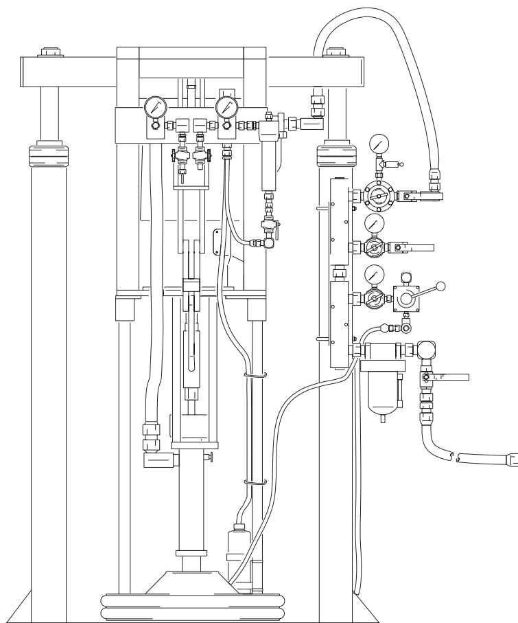
50:1 King Pump Module Shown
